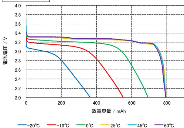
放電温度特性
