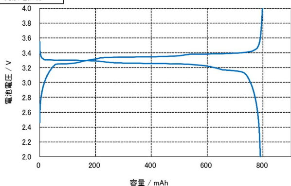
充放電曲線
