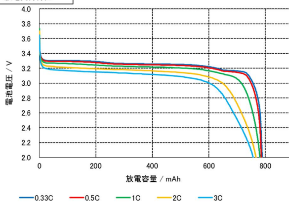
放電負荷特性
