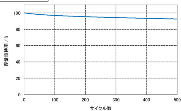
サイクル寿命特性
