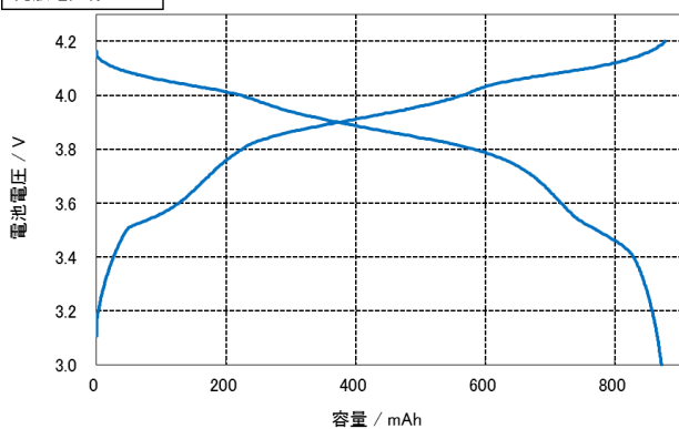
充放電曲線
