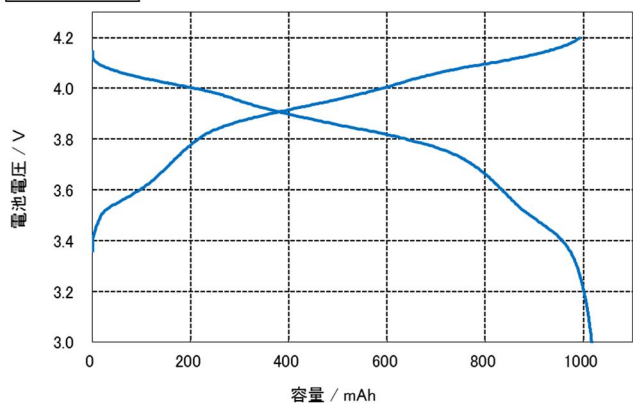
充放電曲線
