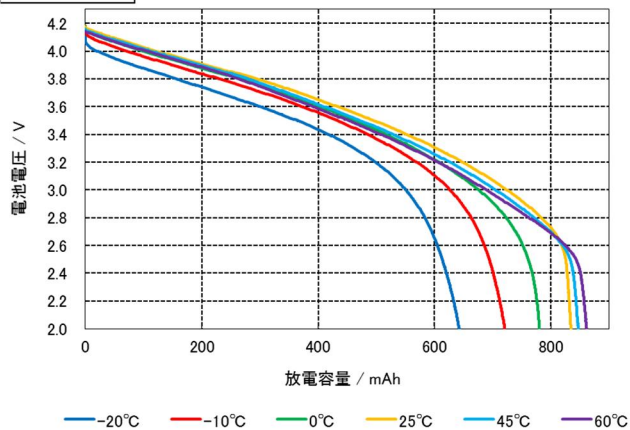
放電温度特性
