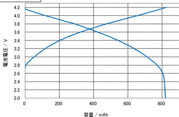
充放電曲線
