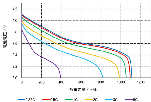
放電負荷特性
