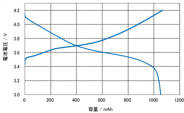
充放電曲線
