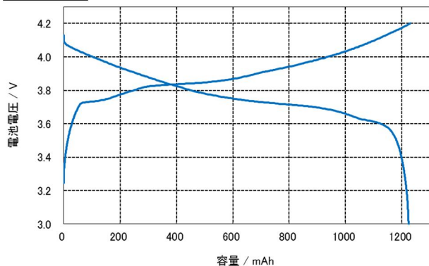
充放電曲線
