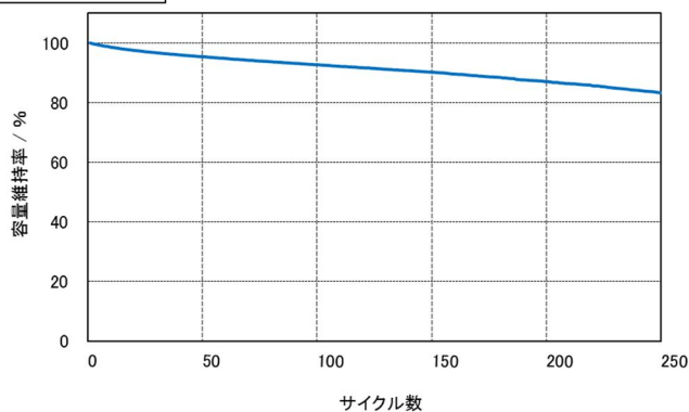
サイクル寿命特性
