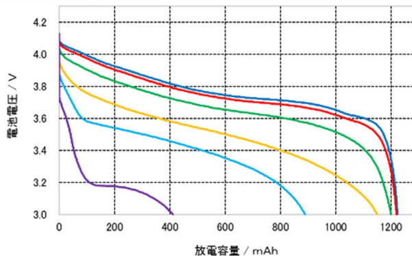
放電負荷特性
